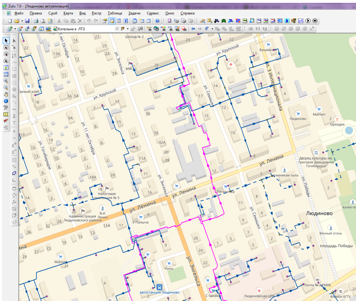
Рисунок 3.1.1. Графическое представление системы теплоснабжения Васильевское сельское поселение с привязкой к топографической основе города с полным топологическим описанием связности объектов
