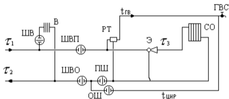
Рисунок 48. Схема подключения потребителей к двухтрубной тепловой сети (при наличии открытой системе теплоснабжения)
