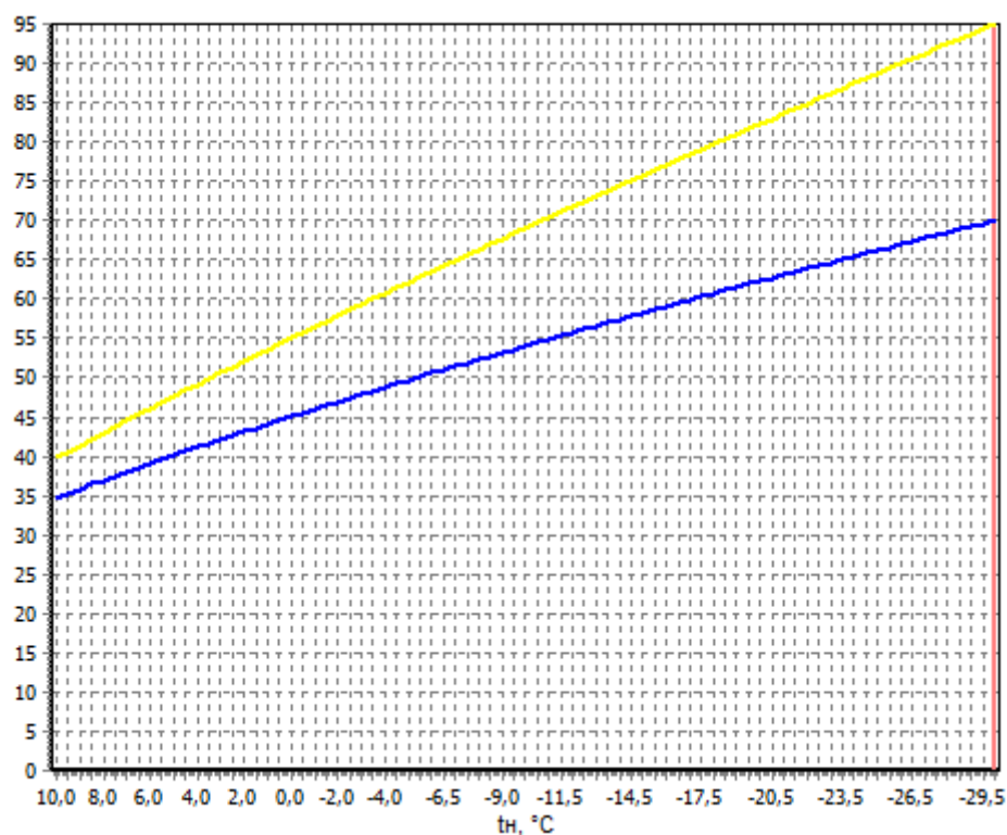
Рис. 1.3.6.2. Температурный график котельной села Китово
