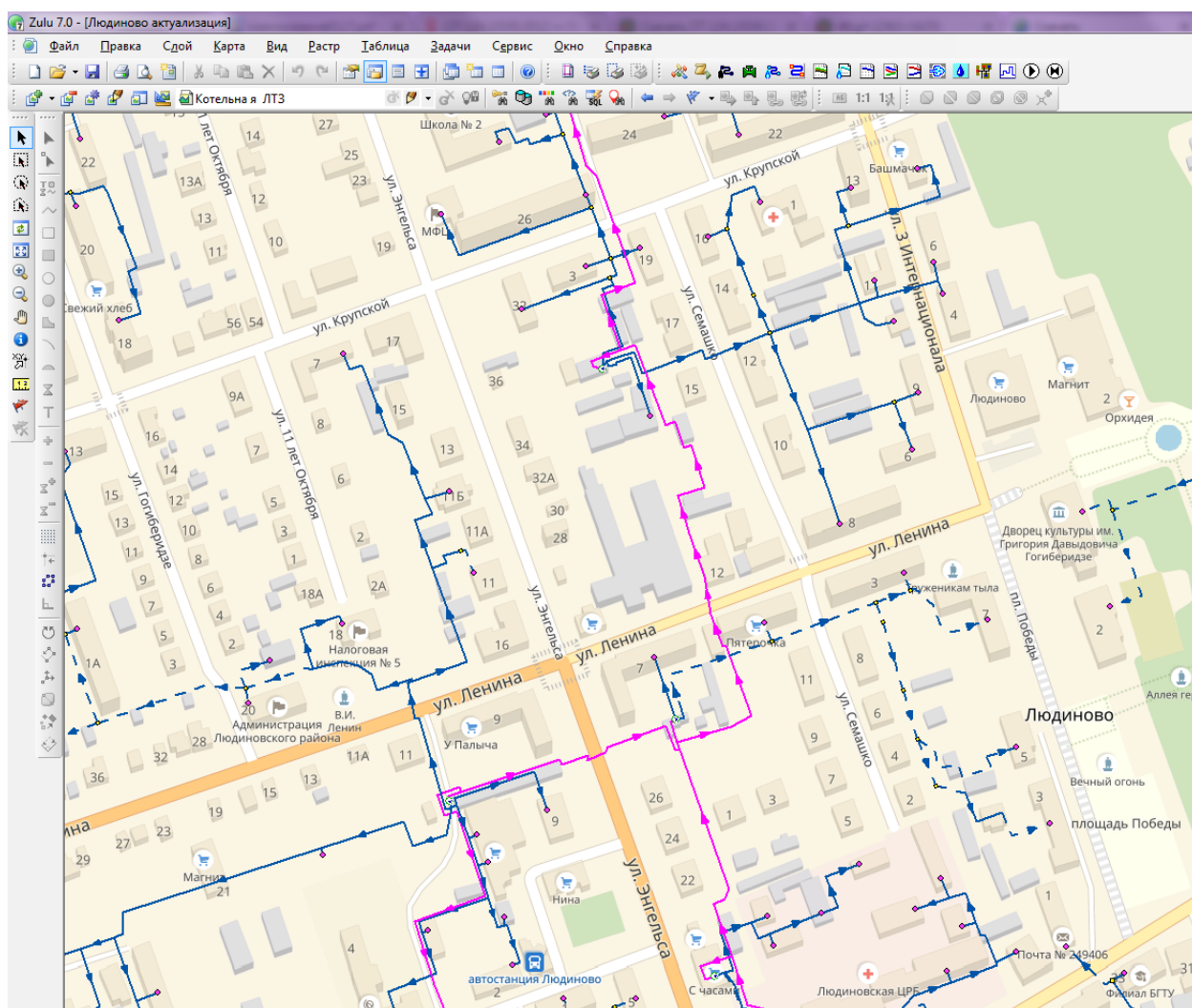
Рисунок 3.1.1. Графическое представление системы теплоснабжения Китовское сельское поселение с привязкой к топографической основе города с полным топологическим описанием связности объектов
