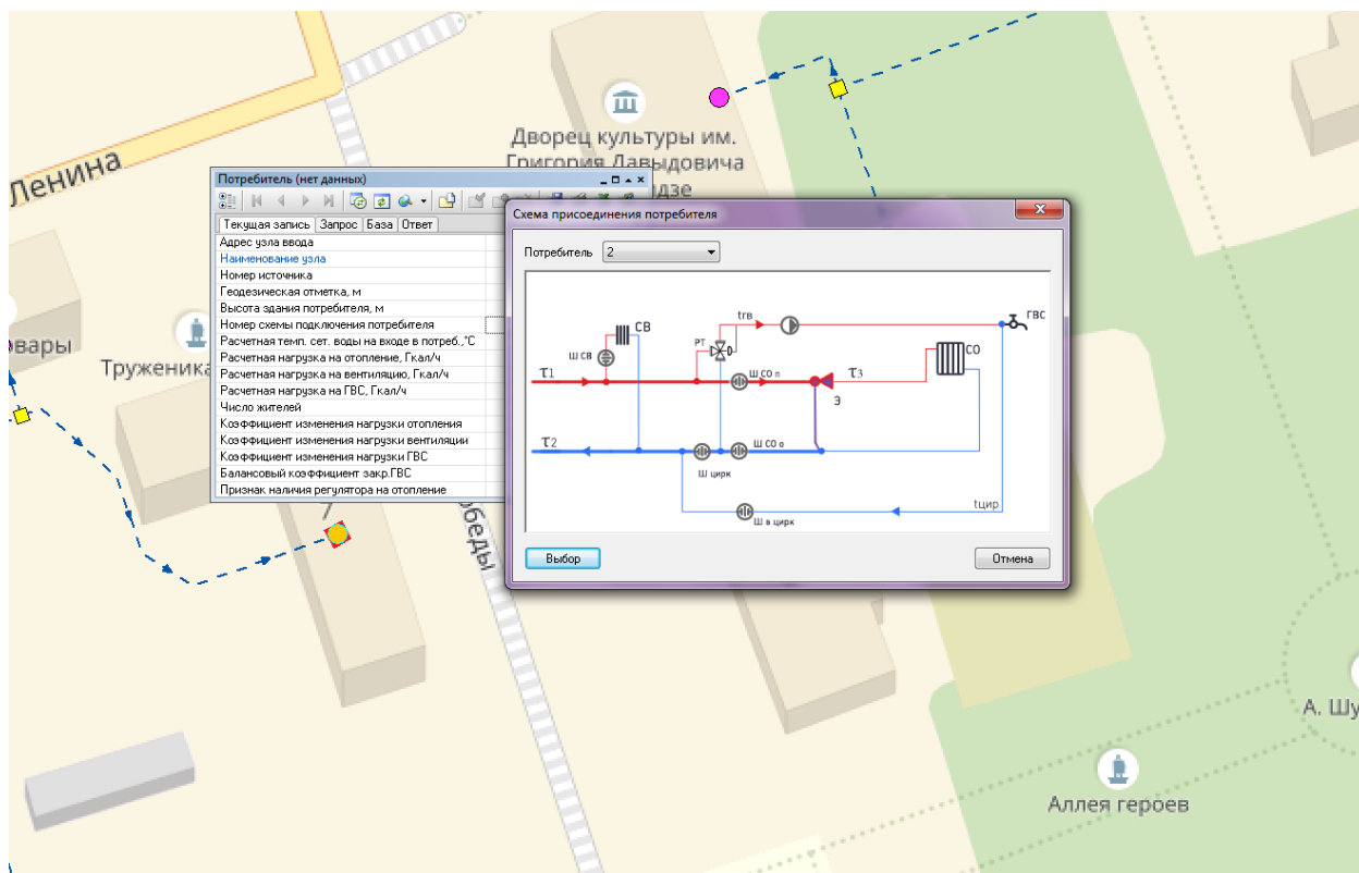
Рисунок 3.2.1. Графическое представление системы теплоснабжения Китовского сельского поселения с привязкой к топографической основе города с полным топологическим описанием связности объектов
