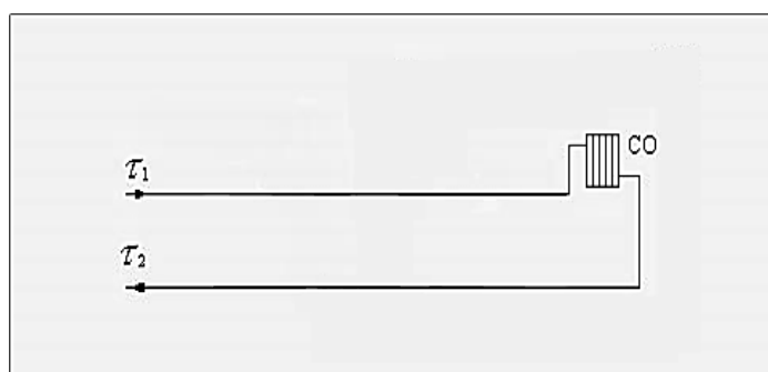
Рисунок 47. Схема подключения потребителей к двухтрубной тепловой сети (при наличии внутридомовой системы отопления)
