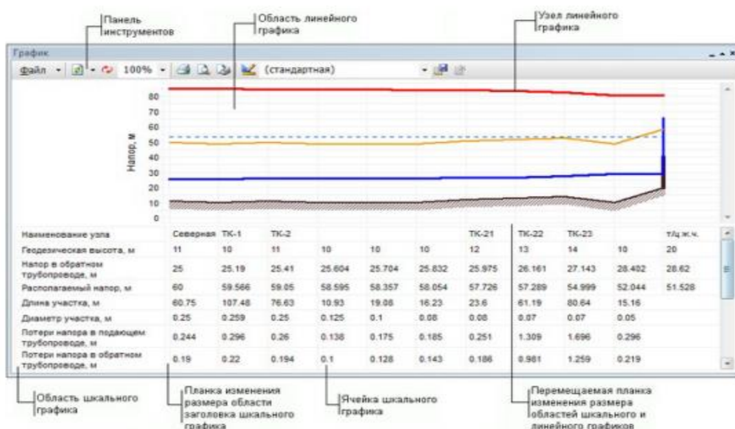
Рисунок 3.9.1. Окно пьезометрического графика
