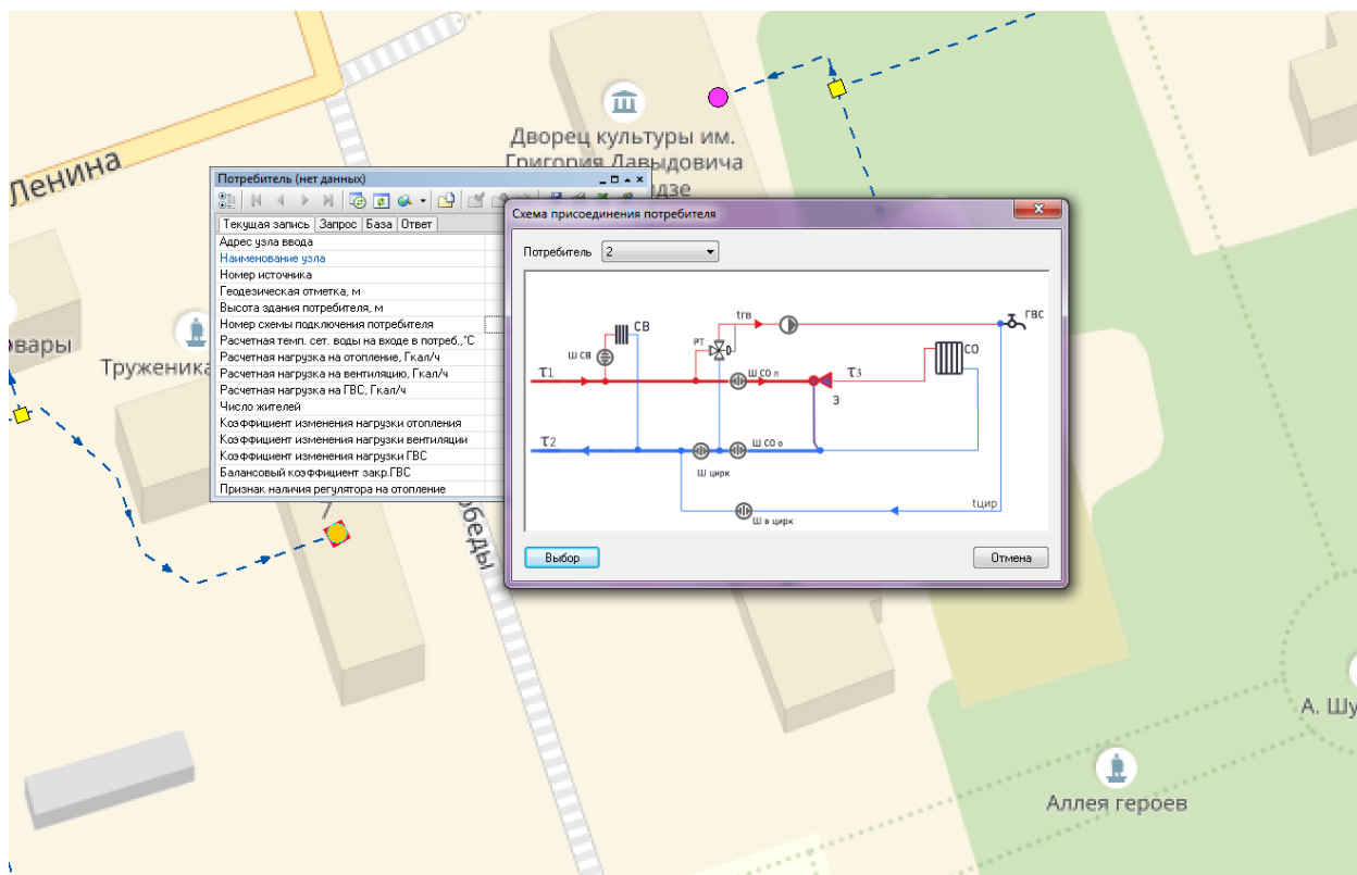
Рисунок 3.2.1. Графическое представление системы теплоснабжения с привязкой к топографической основе с полным топологическим описанием связности объектов
